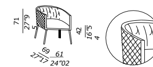
poltroncina - small armchair LOLYTA DUE DIAMOND
