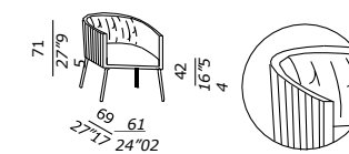
poltroncina - small armchair LOLYTA DUE STRIPE
