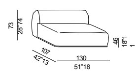
elemento - unit 130
