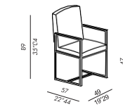
sedia - chair SEI
